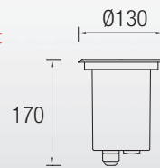
55-9625-CA-37 ■ 1 x G12 150W HID >80°C IP 67 IK 08
