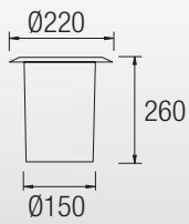
55-9187-CA-37 ■ 1 x G12 70W HID >80°C IP 67 IK 08
