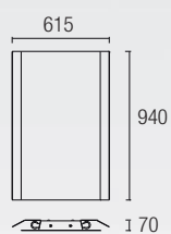
75-4371-K3-M1 2 x T5 39W
