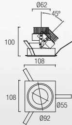
90-3477-14-14 LED CREE max. 8,8W 646 Lm lm 3000 K
