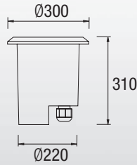
55-9625-CA-37 ■ 1 x G12 150W HID >80°C IP 67 IK 08
