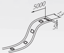
91-2491-00-00 LED 36W 820 Lm lm RGB
